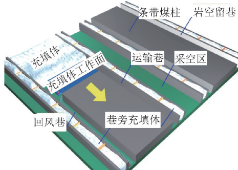
(b) 回采条带煤柱的充填工作面
