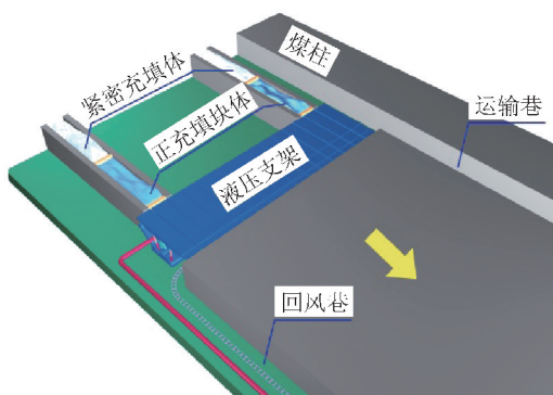
图4 巷旁分段充填示意
