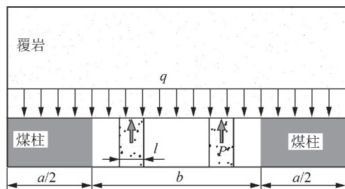
图3 充填体支承压力模型
