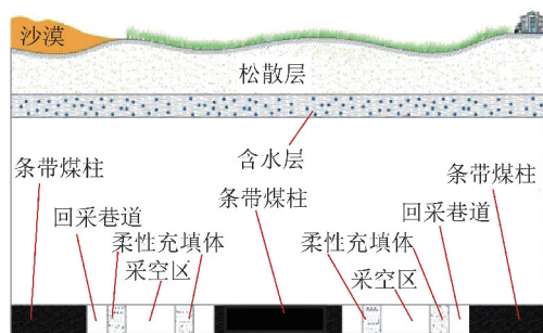
(a) 巷旁充填岩空留巷
