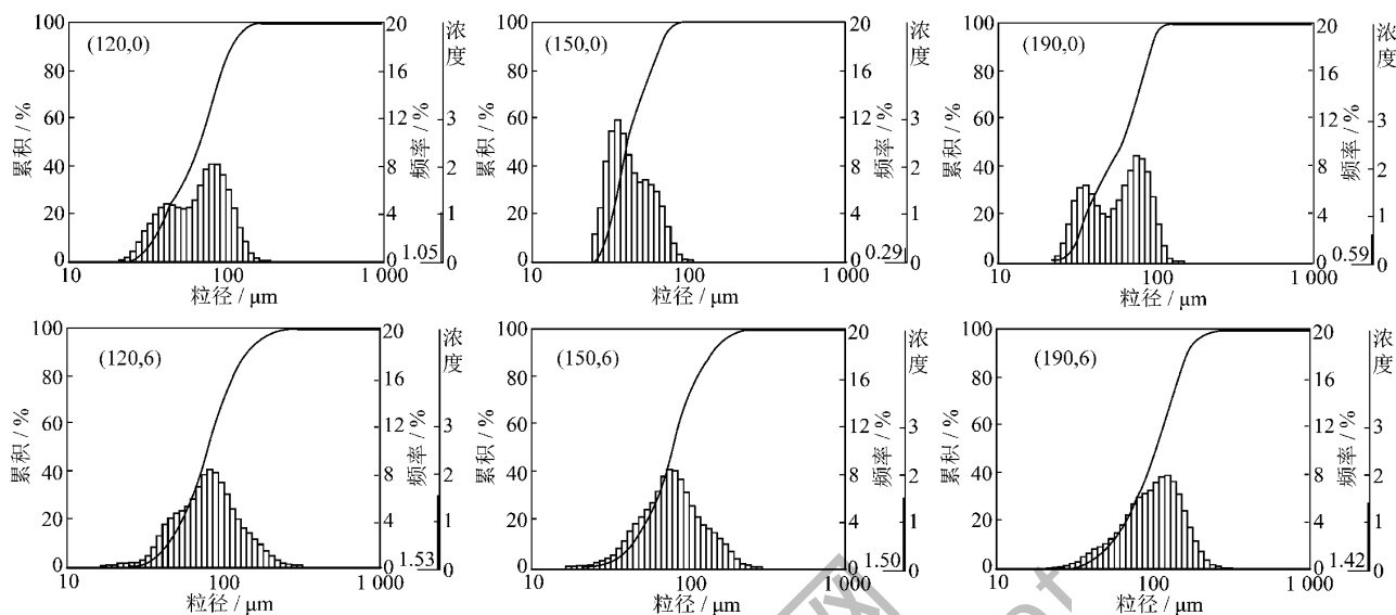
图 3 雾场粒径分布分析 (8 MPa)
