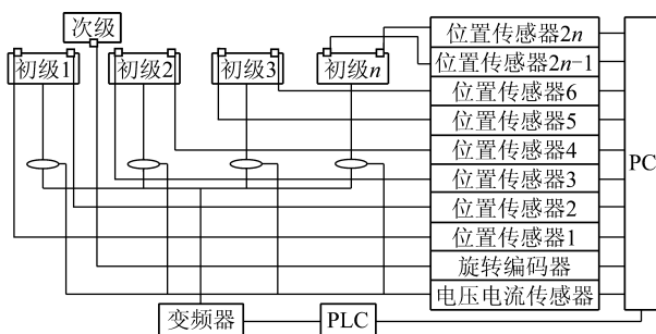
图2 试验系统
