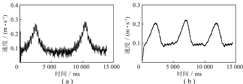
图4 失电后电机动子的仿真速度和试验速度
