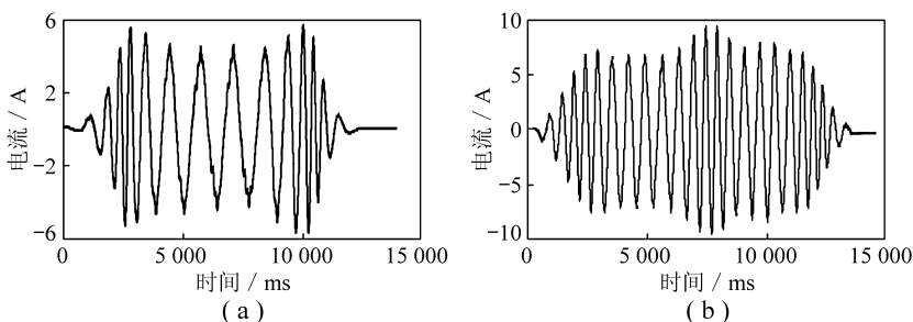
图3 发电制动过程中c相绕组短接时流过的仿真电流(a)和试验电流(b)
