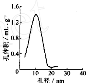
图 2 AI-MFI 型吸附剂的孔径分布曲线
