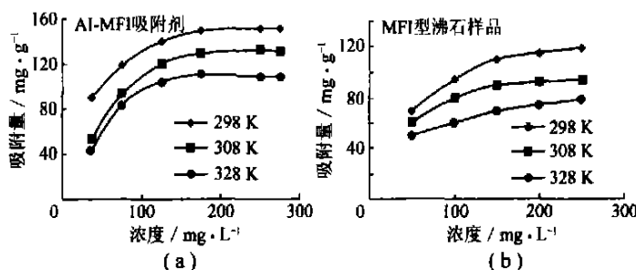
图 4 AI-MFI 吸附剂和 MFI 型沸石样品的苯酚吸附等温线
