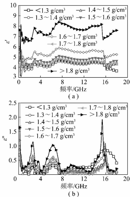
图 5 各密度级煤样的介电性质
