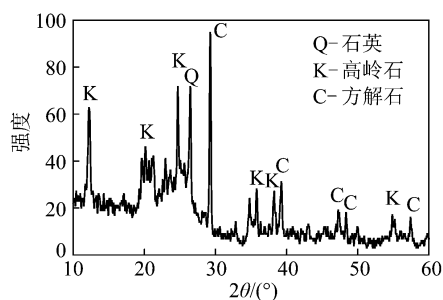
图 2 原煤 XRD 图谱
