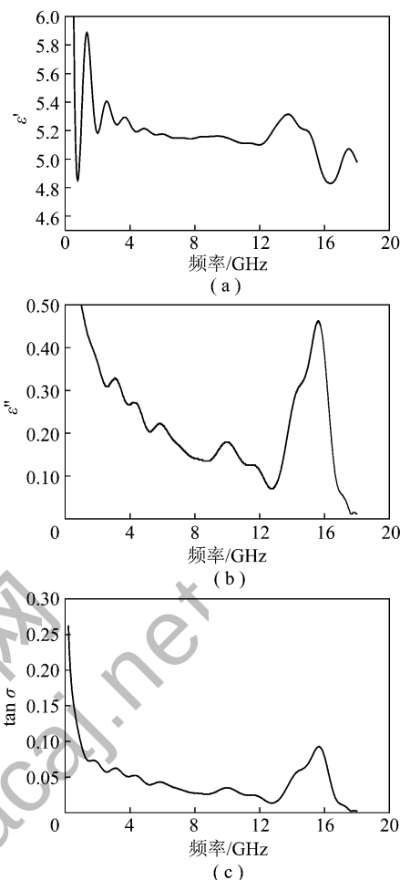
图 1 原煤介电性质
