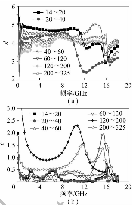
图4 各粒度级煤样的介电性质
