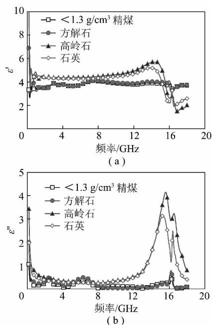
图3 矿物质对介电性质的影响
